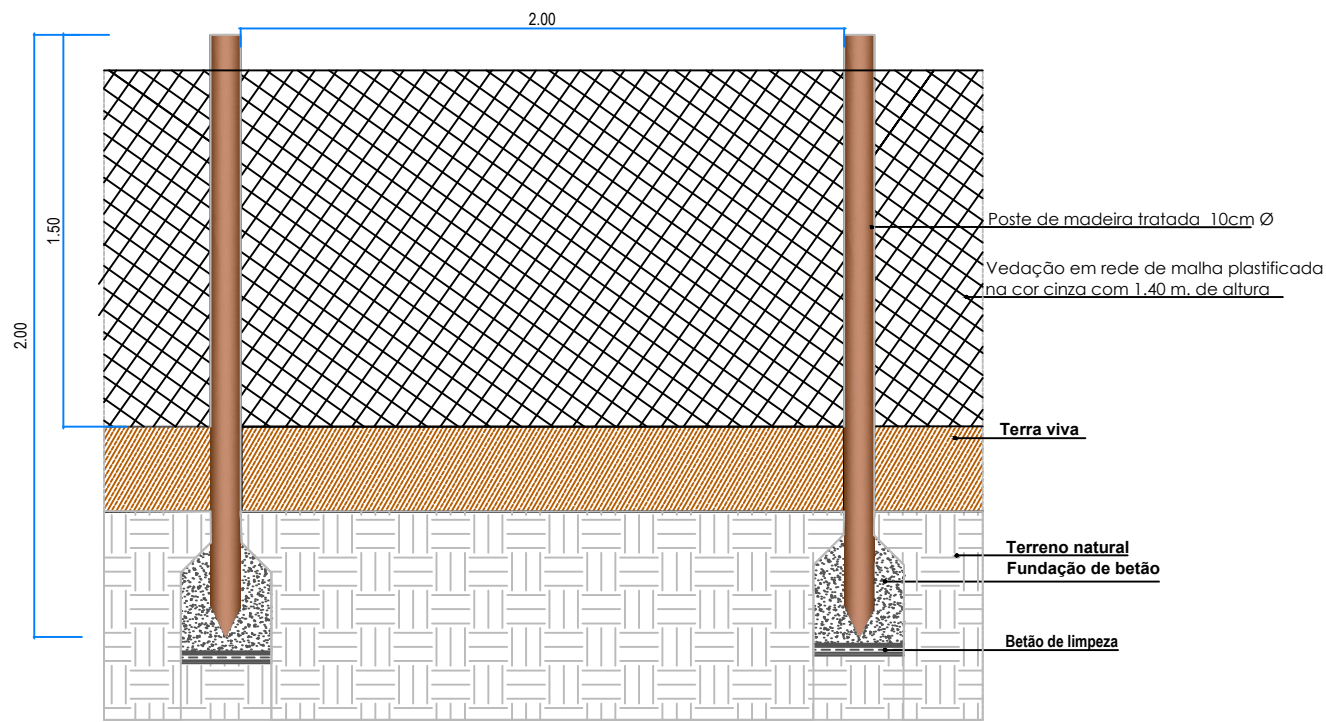
P - PORMENOR DA VEDAÇÃO EM REDOR DOS TALHÕES HORTÍCOLAS ESC.1/20
