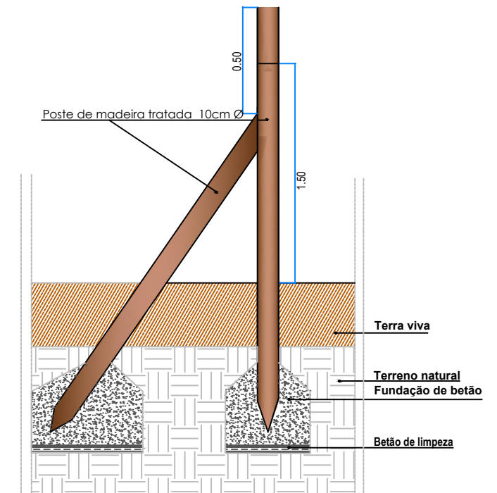
P - PORMENOR DO SISTEMA DE TRAVAMENTO DA VEDAÇÃO NOS CANTOS
