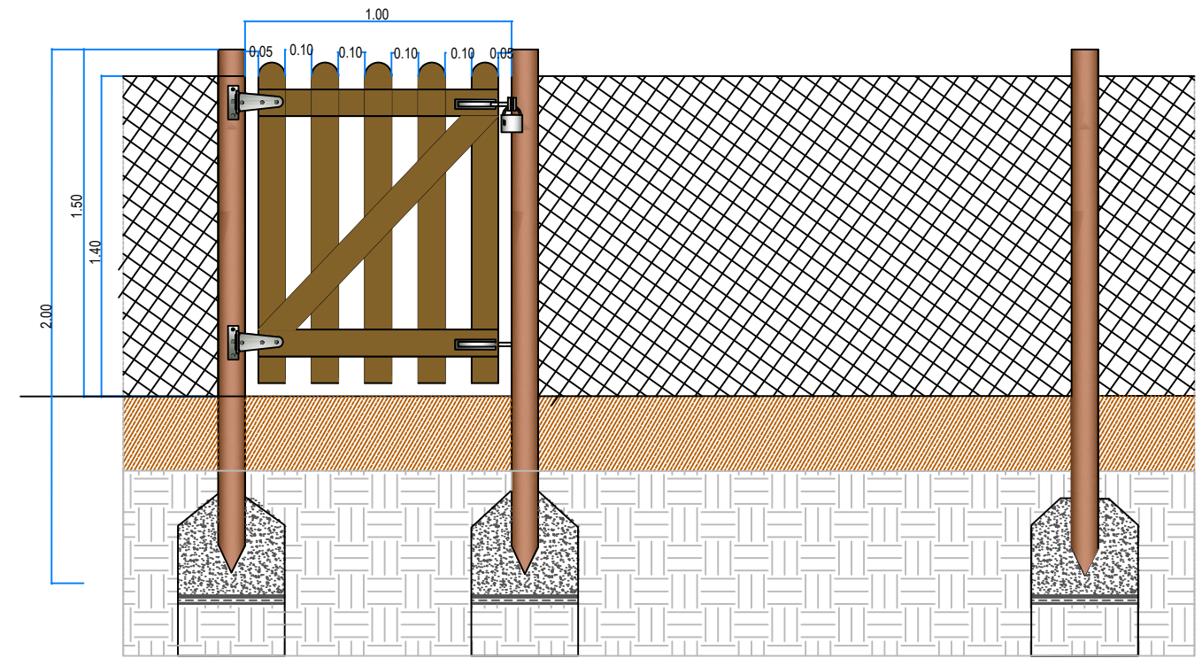
P - PORMENOR DA VEDAÇÃO E PORTÃO DOS TALHÕES HORTÍCOLAS
