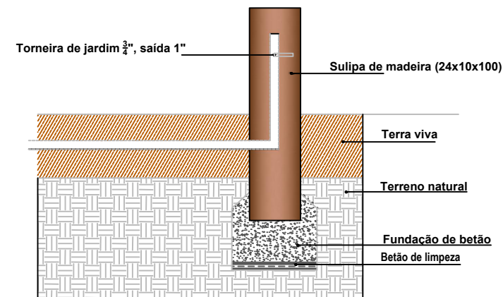
P - PORMENOR DA INSTALAÇÃO DO ABASTECIMENTO DE ÁGUA ÀS HORTAS
