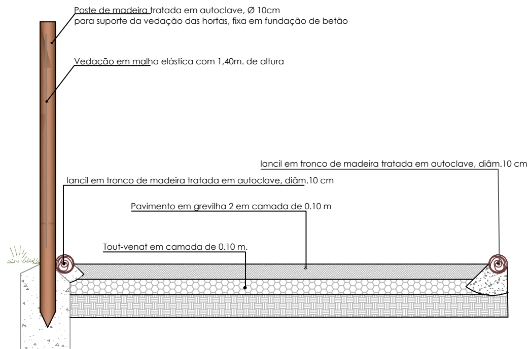
Pormenor dos caminhos nas hortas P - PORMENOR DO PAVIMENTO EM GREVLHA ESC.1/20
