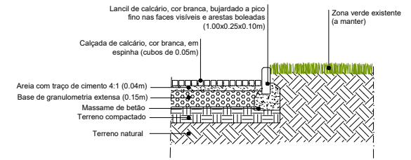
P5 - Remate entre caminho em calçada de calcário e zona verde existente
