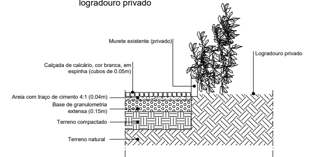
P7 - Remate entre caminho em calçada de calcário e logradouro privado
