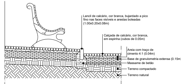
P6 - Remate entre caminho em calçada de calcário e zona com banco, junto ao edifício
