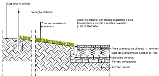
P3 - Remate entre caminho em calçada de calcário, zona verdee logradouro privado
