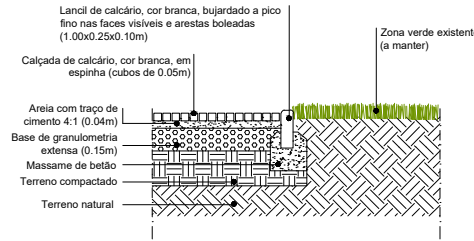
P4 - Remate entre caminho em calçada de calcário e zona verde existente (de nível)
