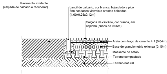
P2 - Remate entre caminho em calçada de calcário e edifício existente
