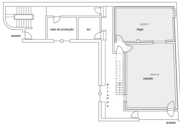
planta - piso 0 - escala 1|100
